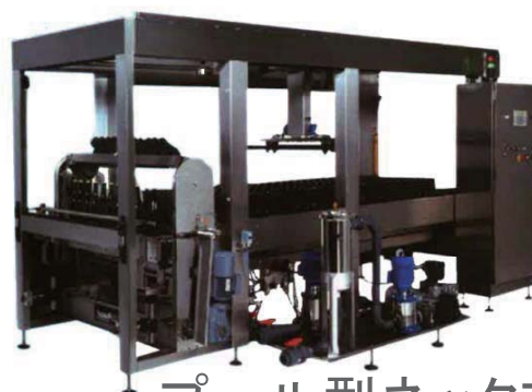
プール型ネックフリーザー (1,200bph~)
