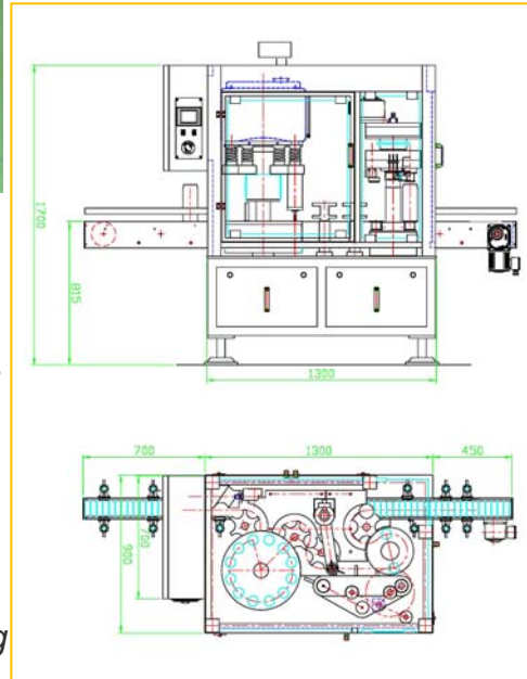
④ 概観図 (TRON 12-2、液体窒素滴下装置のオプション付) 12-head filler, 2-head seamer, TRON 12-2, with LN2 doser option. ⑤ サンプルレイアウト: デパレタイザー → インクジェット → ツストリンサー → TRON12-2 → インバーター → ウォーマー → ウェイトチェッカー → 出口テーブル Sample layout of complete canning line.
