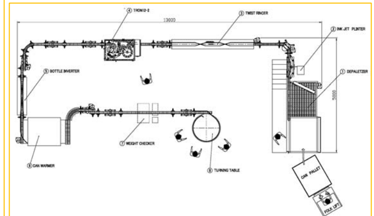
④ 概観図 (TRON 12-2、液体窒素滴下装置のオプション付) 12-head filler, 2-head seamer, TRON 12-2, with LN2 doser option. ⑤ サンプルレイアウト: デパレタイザー → インクジェット → ツストリンサー → TRON12-2 → インバーター → ウォーマー → ウェイトチェッカー → 出口テーブル Sample layout of complete canning line.
