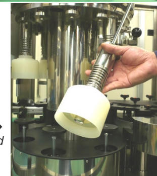
缶用充填ノズル → Gravity filler head
